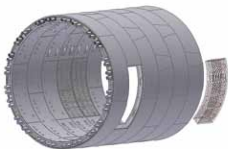
Der Energietübbing wird wie ein normaler Tübbing in die Tunnelchale eingebaut. Benachbarte Energietübbinge werden zu größeren Kreisläufen zusammengeschlossen.
