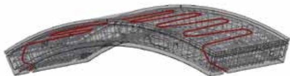
Energietübbing mit innenliegendem Absorberrohr (rot)
