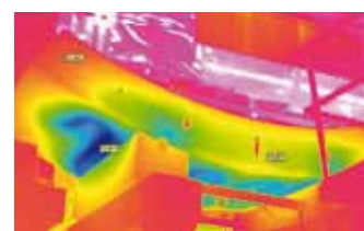
Wärmebild eines Energietübbings im Laborversuch. Deutlich zu erkennen sind die gekühlten Absorberrohre (blau) im Tübbing.
